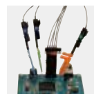
逻辑探头 连接示例
